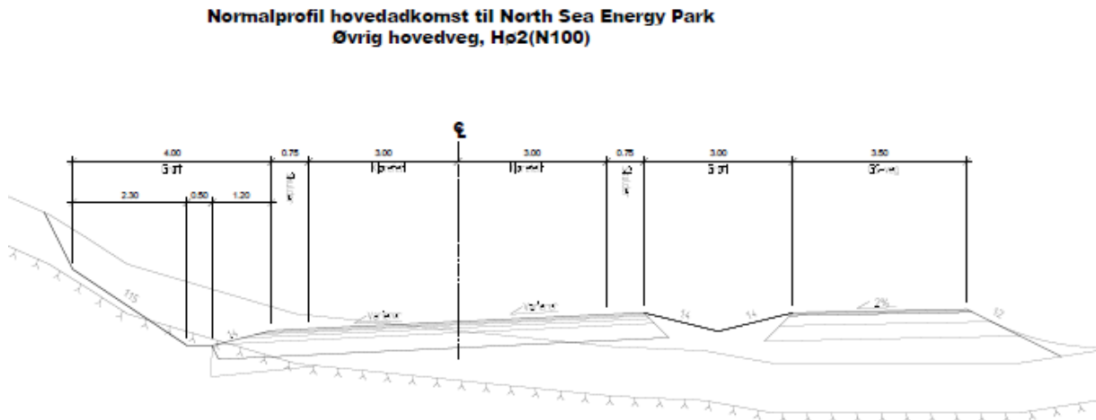
FIGUR 4 NORMALPROFIL HOVEDADKOMSTVEG
