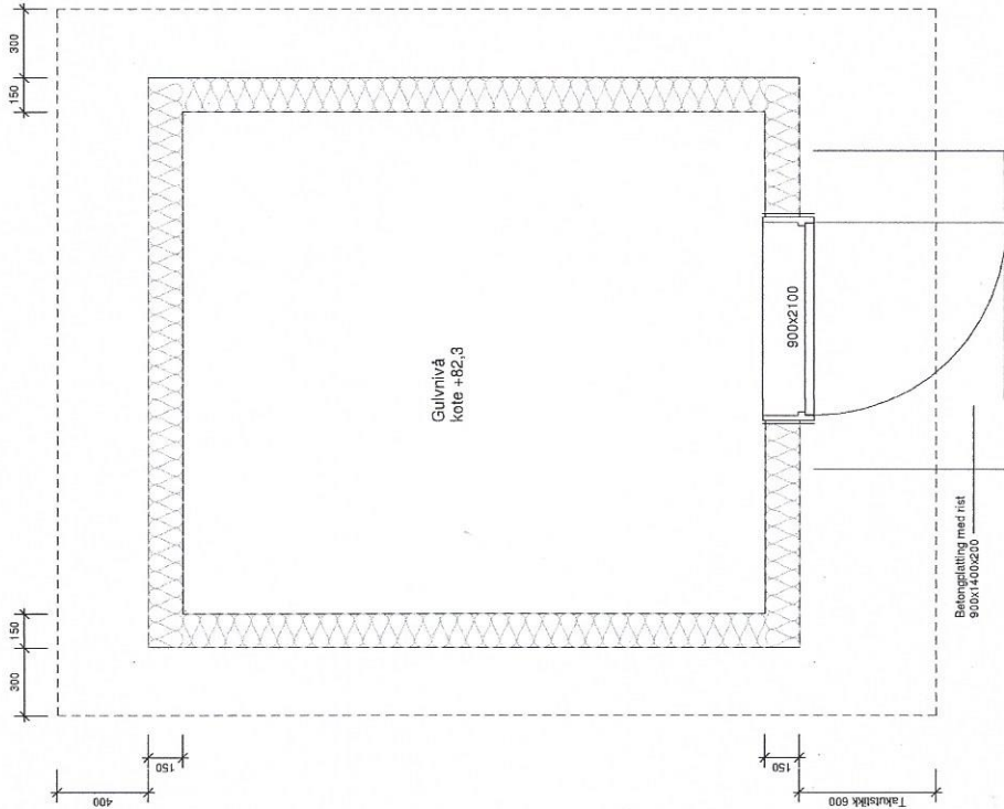
Plan 1 : 25
